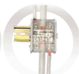
Кріплення на DIN-рейку та монтажну панель
