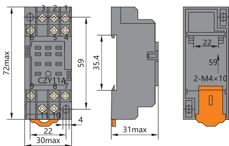
Розетка CZY11A
