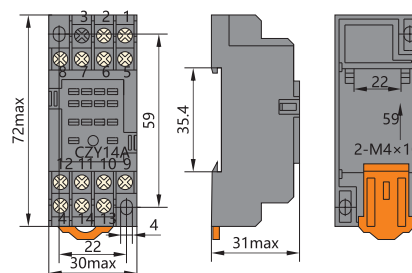
Розетка CZY14A
