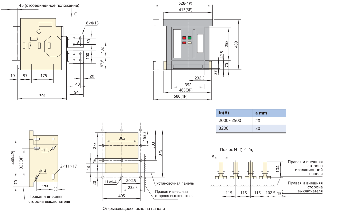
Выключатель выдвижного типа горизонтальный, заднее подсоединение NA1-3200X/NA1-3200XN
