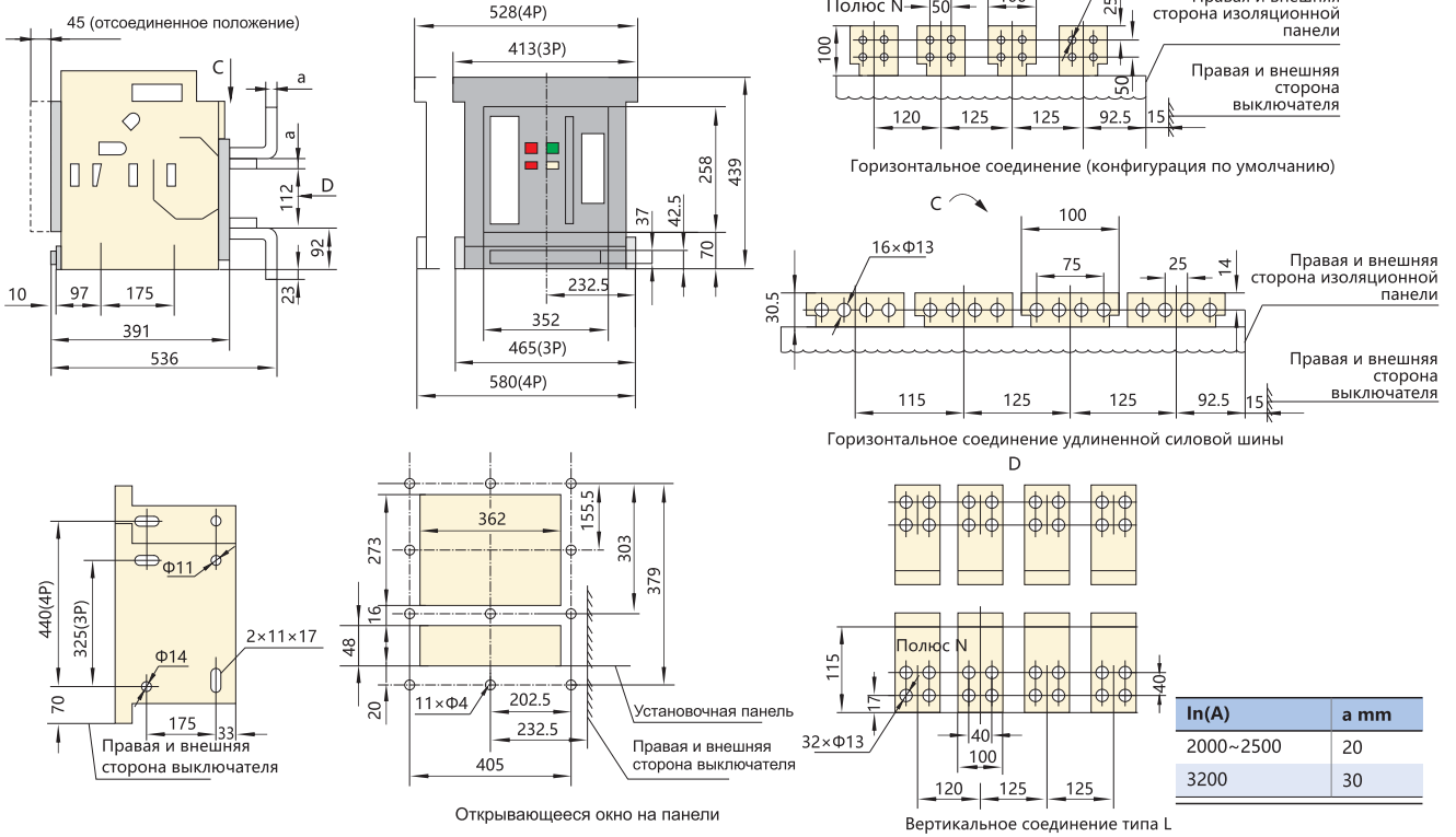
Выключатель выдвижного типа горизонтальный, заднее подсоединение NA1-3200X/NA1-3200XN
