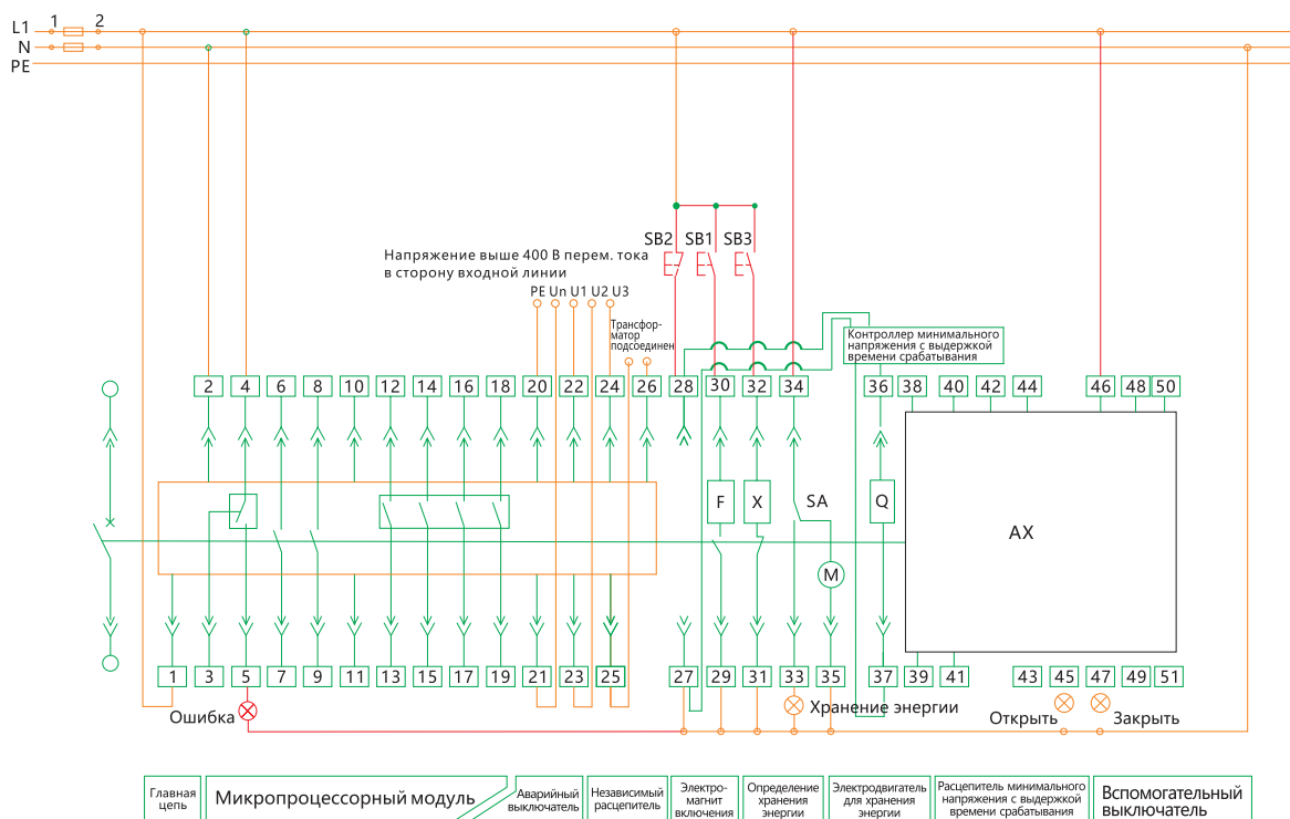
Вторичная схема микропроцессорного блока типа 3М NA1-2000X~6300X (с расцепителем минимального напряжения с задержкой)
