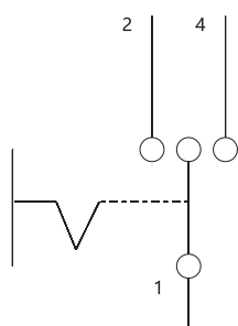
NZK1-32/1
