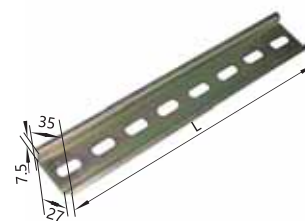
Размеры монтажной рейки
