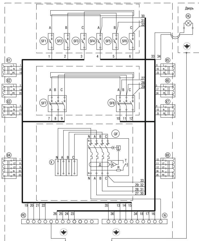
Рисунок 1 – Схема электрическая
