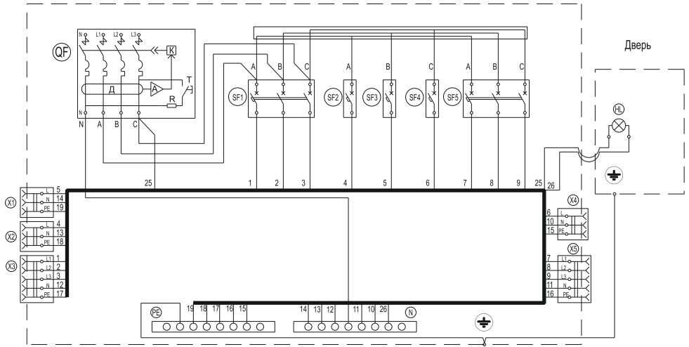
Рисунок 1 – Схема электрическая
