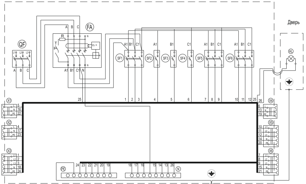
Рисунок 1 – Схема электрическая
