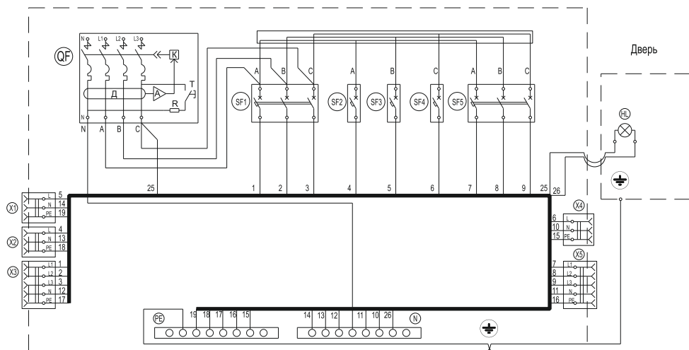
Рисунок 1 – Схема электрическая
