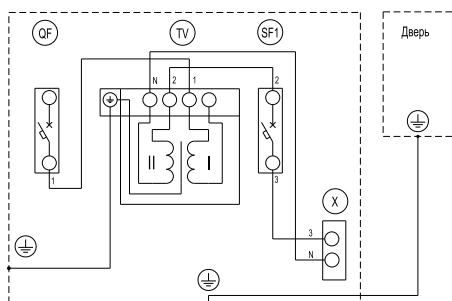
Рисунок 1 – Схема электрическая ящика ЯТП-0,25 230/42-2 УХЛ2 IP54
