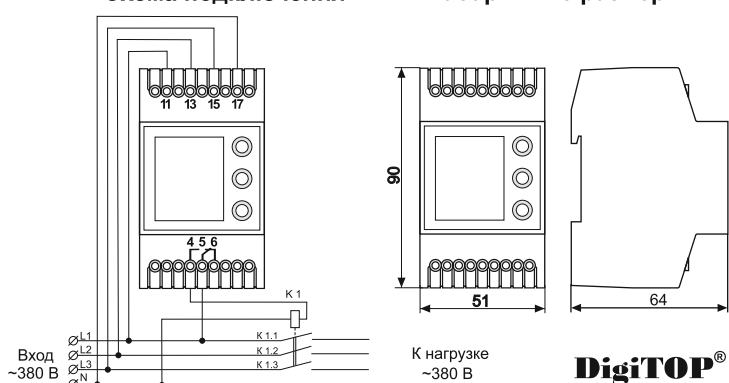
Схема подключения
