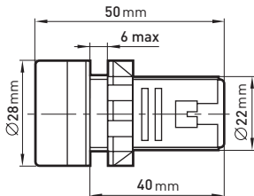
Габаритні розміри e.ad22.am, e.ad22.va e.ad22.fr, e.ad22.temp
