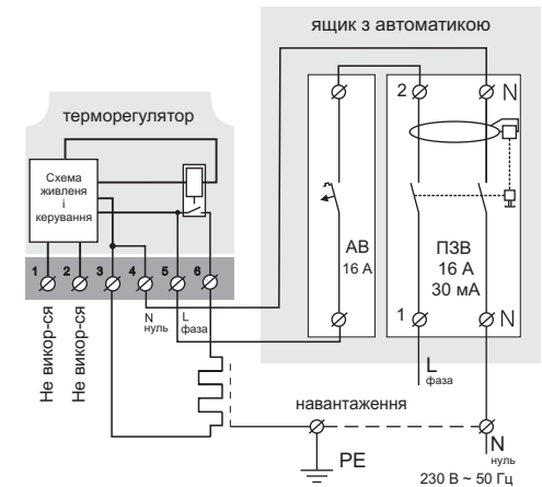
Схема 2. Підключення автоматичного вимикача і ТЗВ
